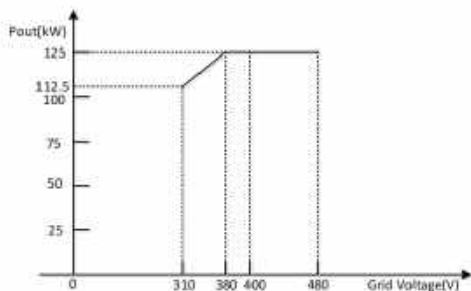
SOFAR 125KTLX-G4 Krzywa spadku parametrów znamionowych zależnie od napięcia AC (Pf=1)
