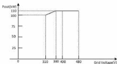
SOFAR 110KTLX-G4 Krzywa spadku parametrów znamionowych zależnie od napięcia AC (Pf=1)
