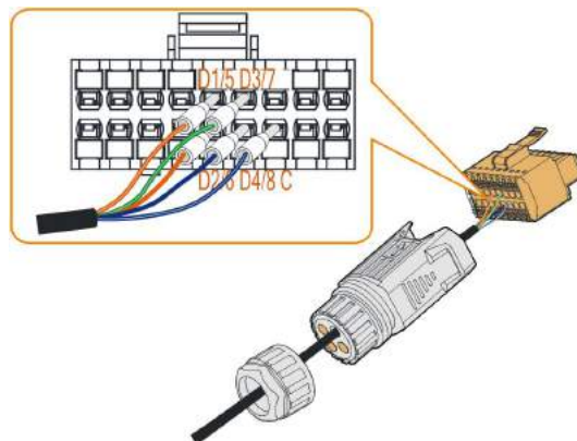
Rys. 5-10 Połączenie DI
