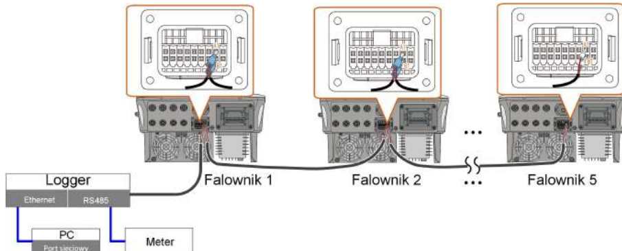
Rys. 5-6 Podłączanie wielu falowników
