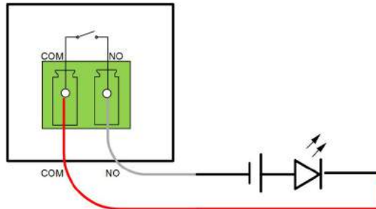
Rys. 5-9 Styk DO normalnie otwarty
