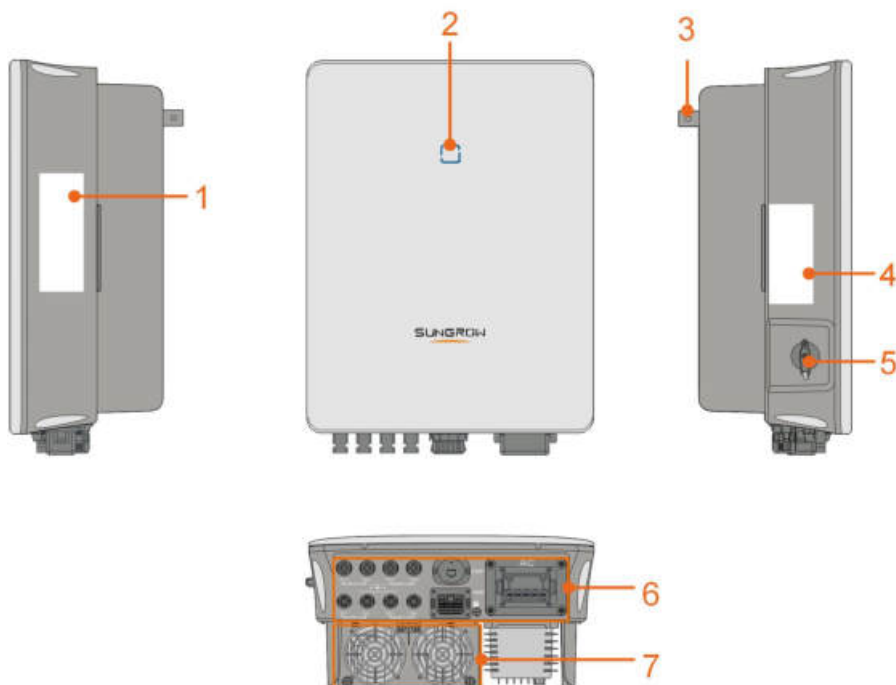
Rys. 2-2 Wygląd falownika
