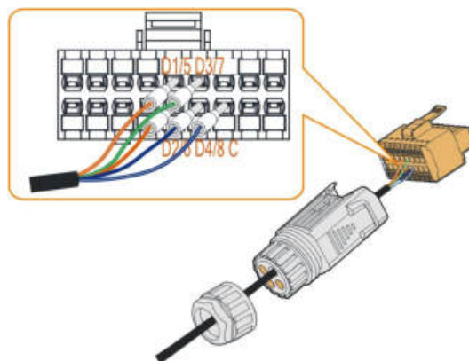
Rys. 5-10 Połączenie DI
