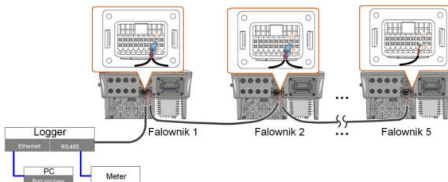
Rys. 5-6 Podłączanie wielu falowników
